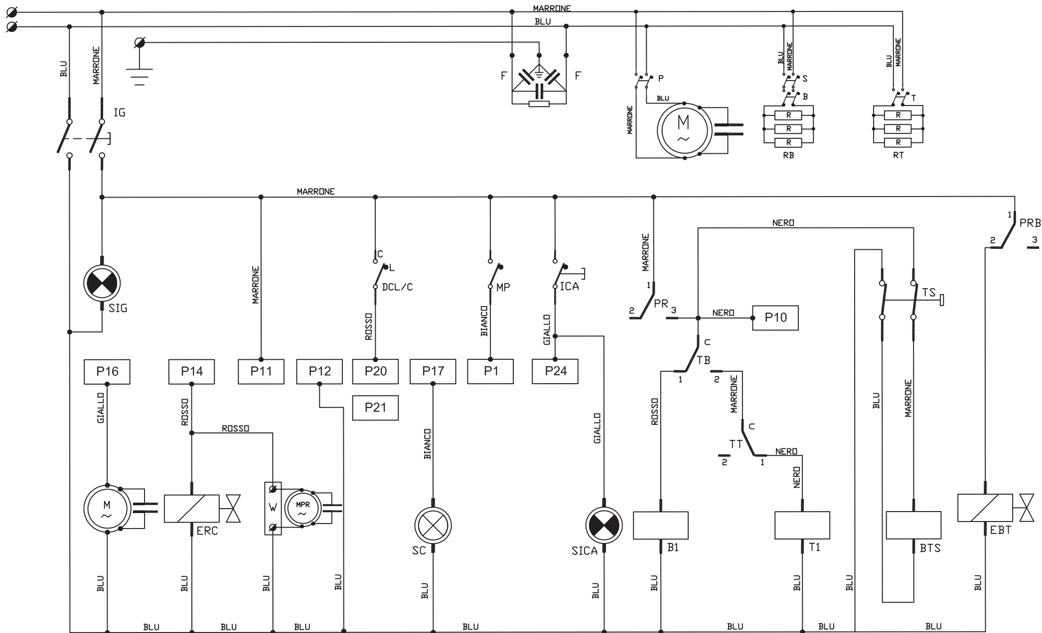
COMPACT- Breaktank - 230V~50Hz sez. Ø 3x4 con timer elettronico Serial # 85069 onwards
